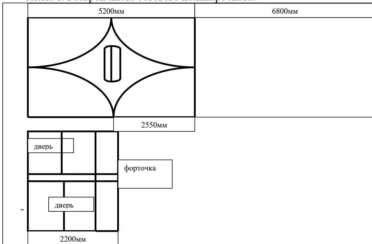
Схема 1. Раскрой листа сотового поликарбоната.
